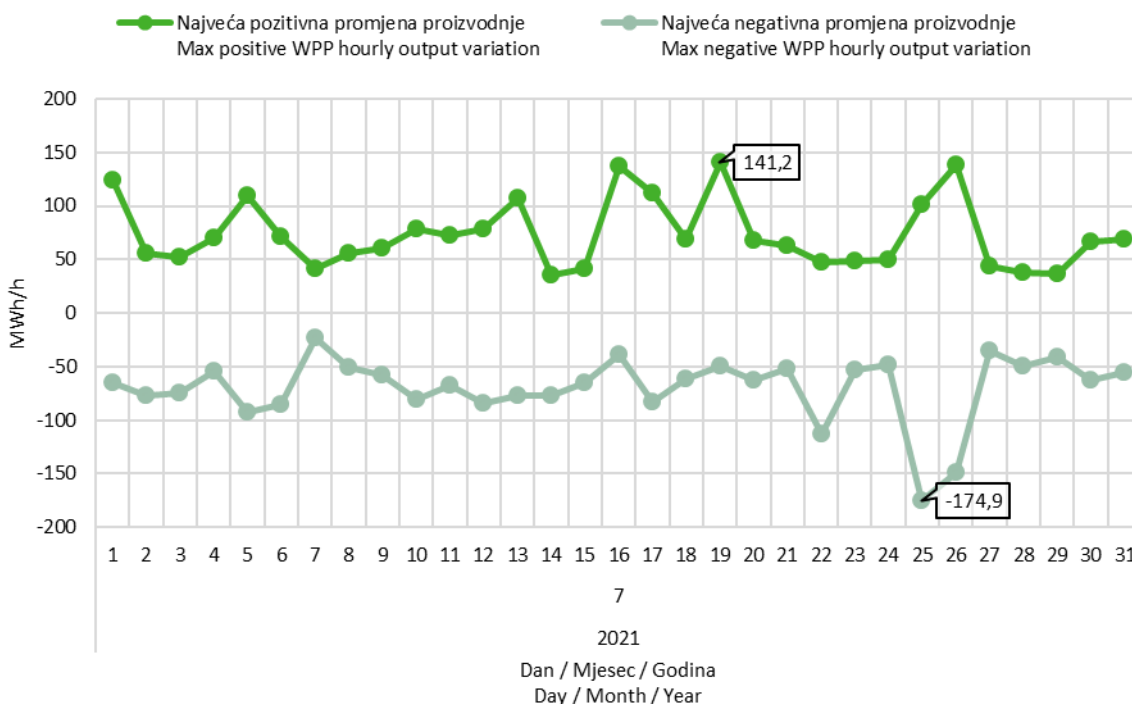
Slika 9 Maksimalna pozitivna i maksimalna negativna promjena satne proizvodnje VE u srpnju 2021. godine
