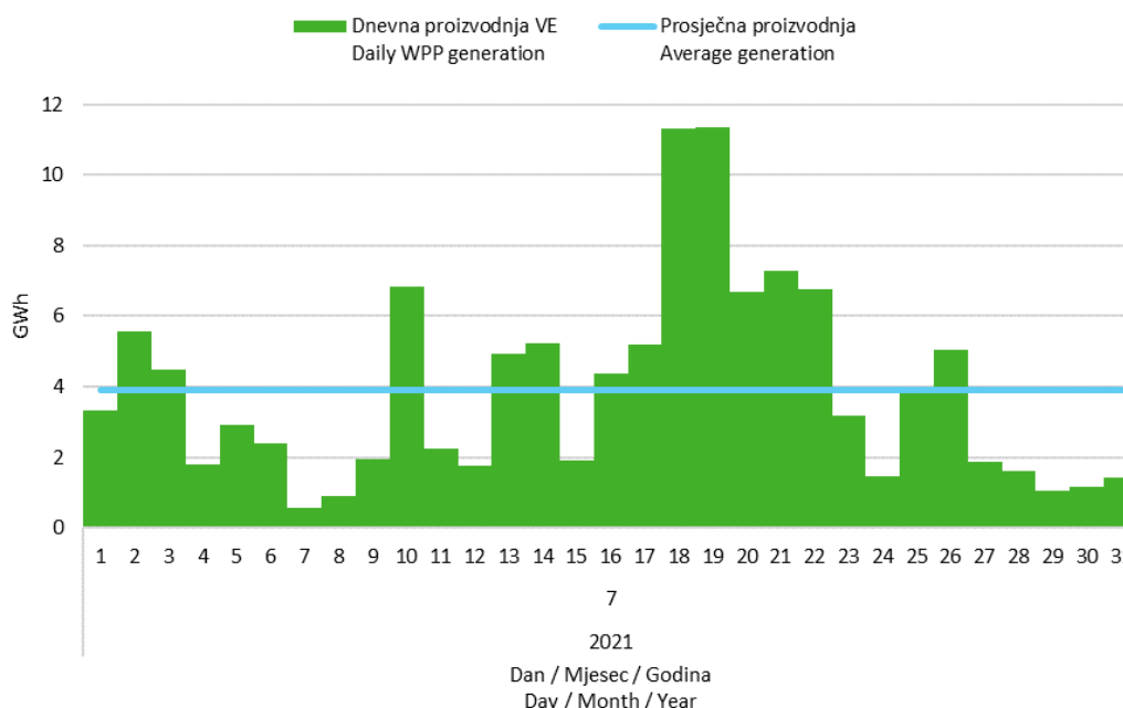
Slika 5 Dnevna proizvodnja svih vjetroelektrana u srpnju 2021. godine
