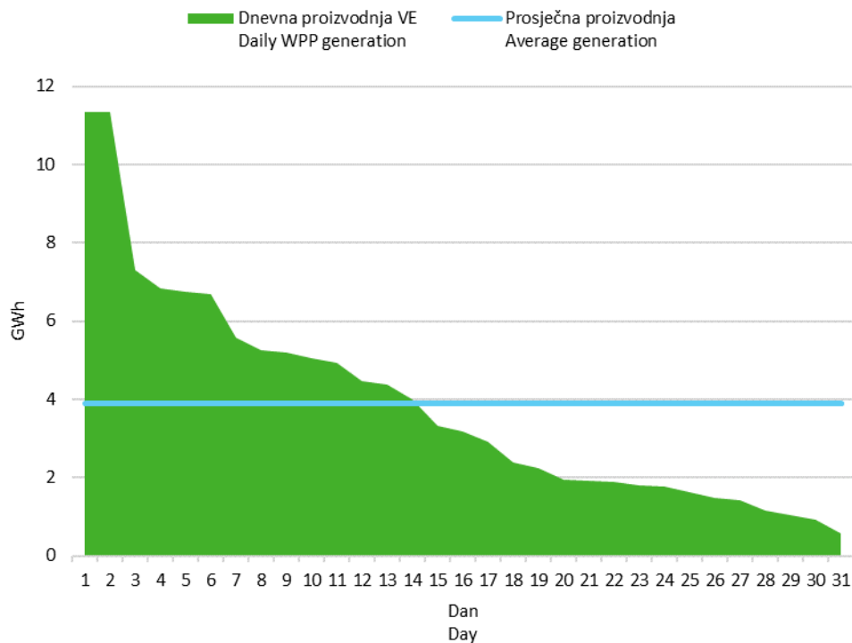
Slika 6 Krivulja trajanja dnevne proizvodnje vjetroelektrana u srpnju 2021. godine
