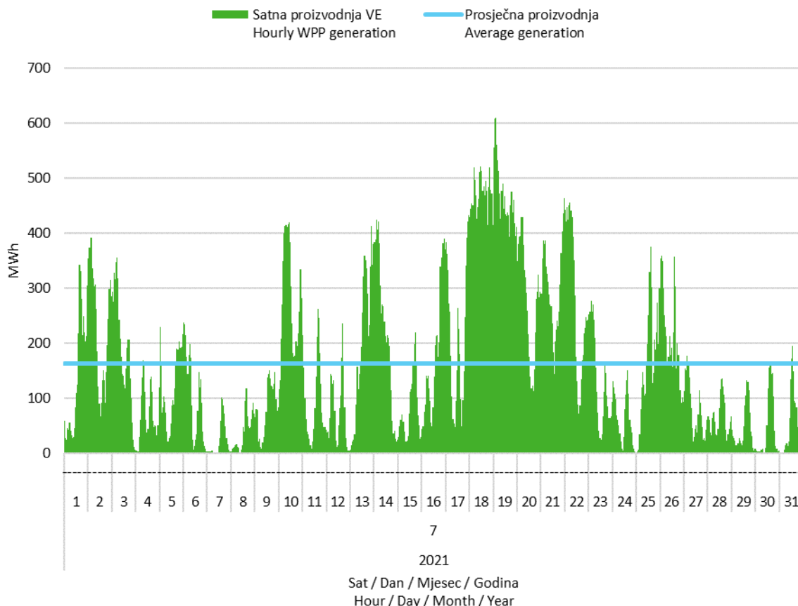
Slika 2 Satna proizvodnja svih vjetroelektrana u srpnju 2021. godine
