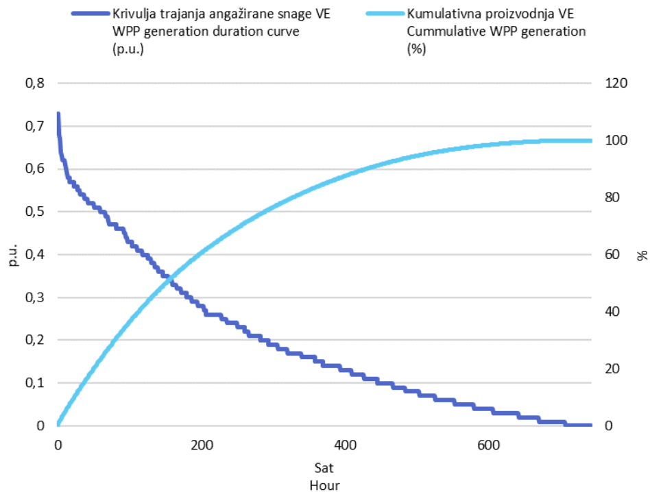
Slika 3 Krivulja trajanja angažirane snage svih VE i kumulativna proizvodnja VE u srpnju 2021. godine u jediničnim vrijednostima
