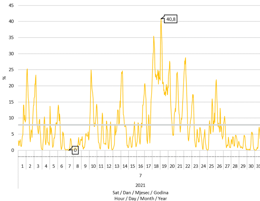
Slika 8 Udio proizvodnje vjetroelektrana u pokrivanju satnog opterećenja elektroenergetskog sustava u srpnju 2021. godine
