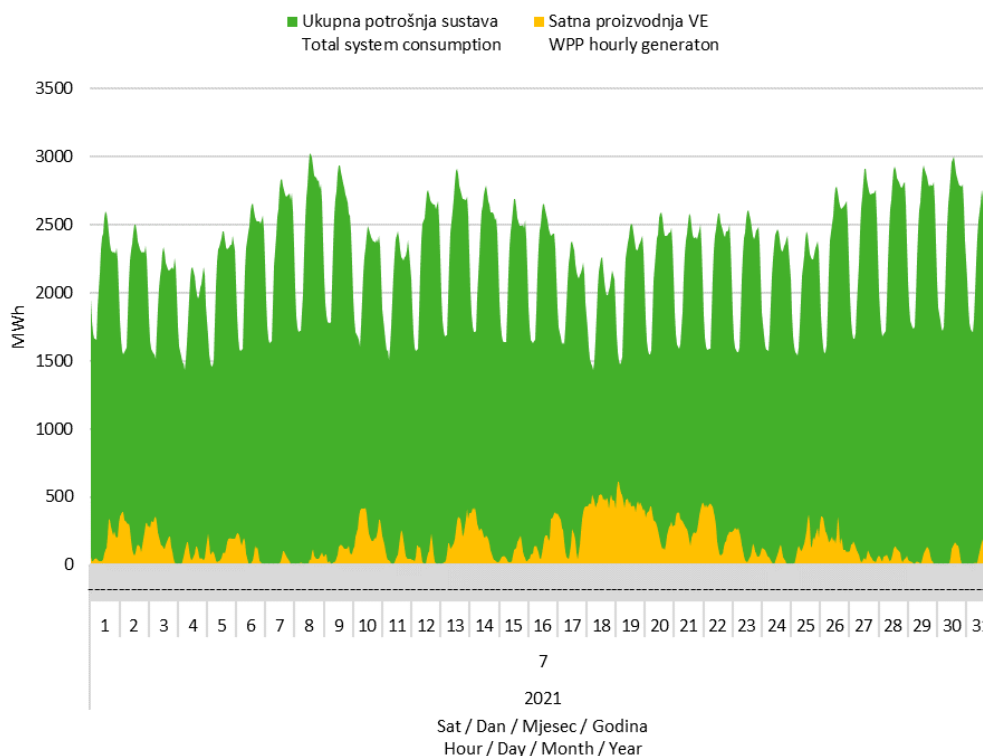
Slika 7 Usporedba satnog dijagrama opterećenja sustava i proizvodnje vjetroelektrana u srpnju 2021. godine
