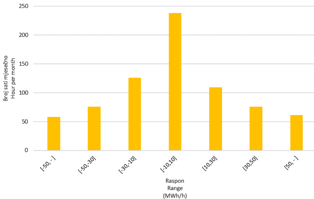
Slika 10 Statistička raspodjela satnih promjena proizvodnje VE u srpnju 2021. godine
